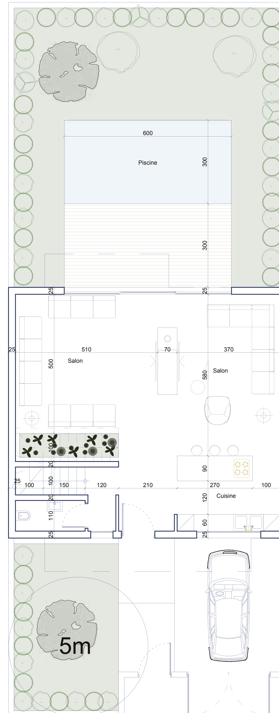
Rez De Chaussee Surface 90 M 2
