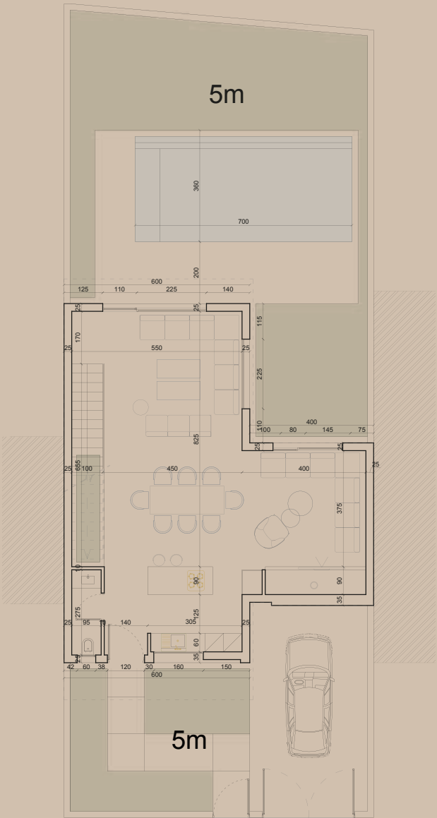
Rez-de-chaussée
