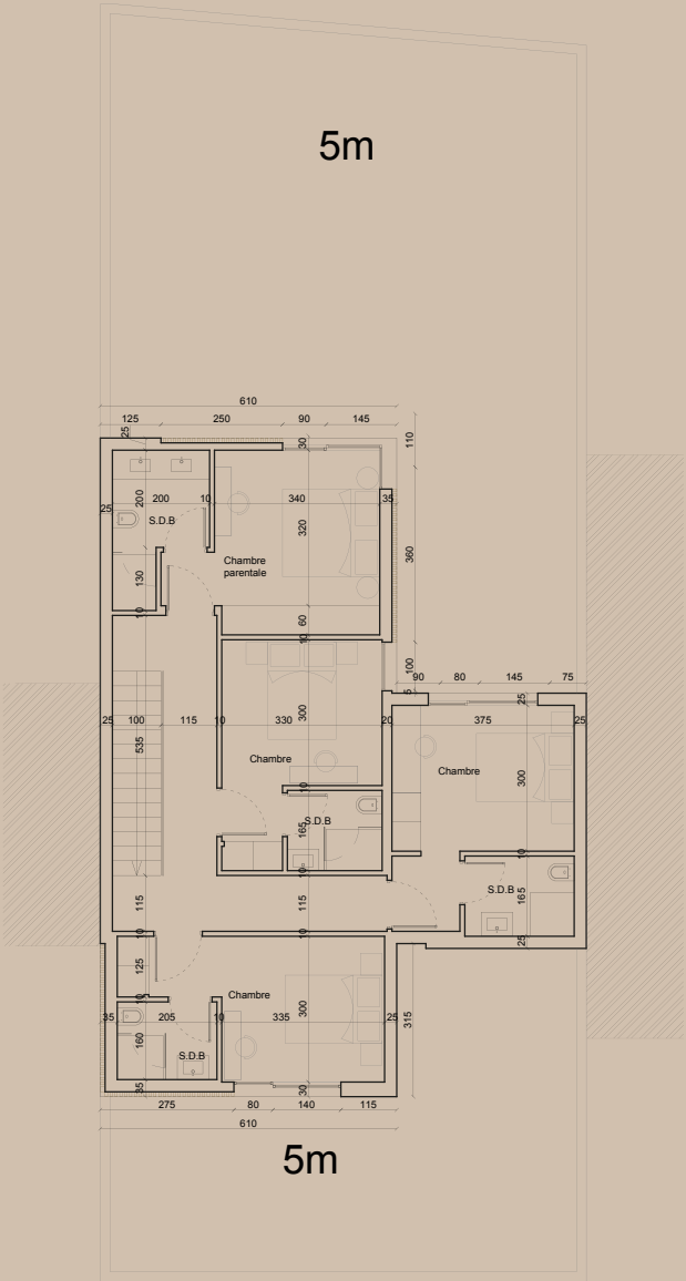
Etage
