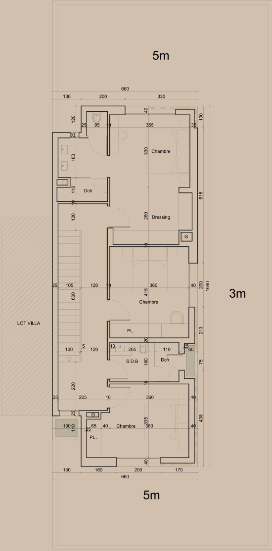
Etage
