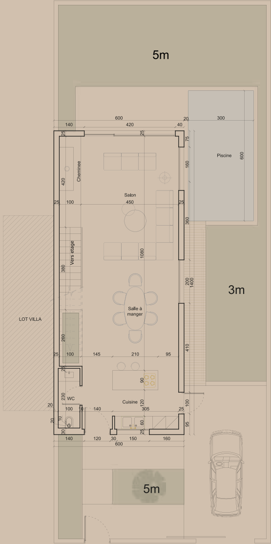
Rez-de-chaussée
