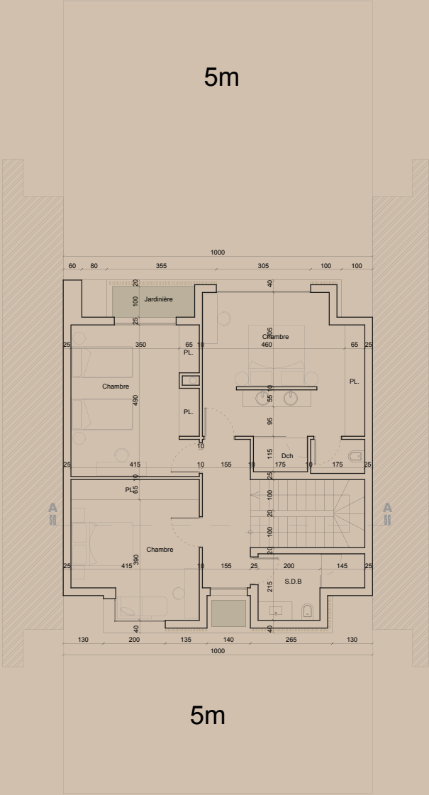
Etage
