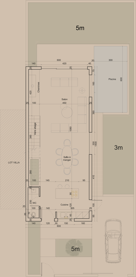
Rez-de-chaussée
