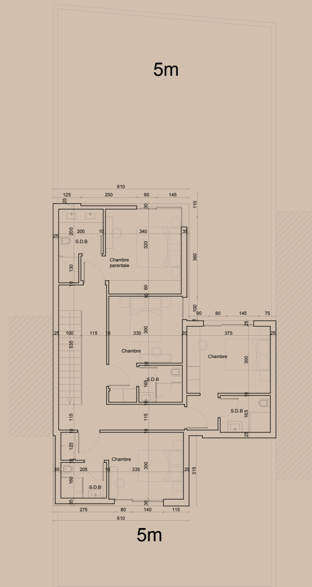
Etage
